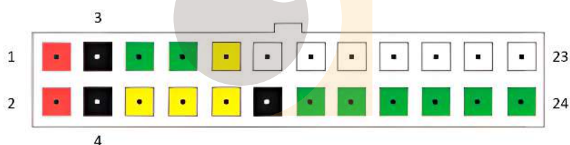
Рисунок 3 – Интерфейсный разъём
