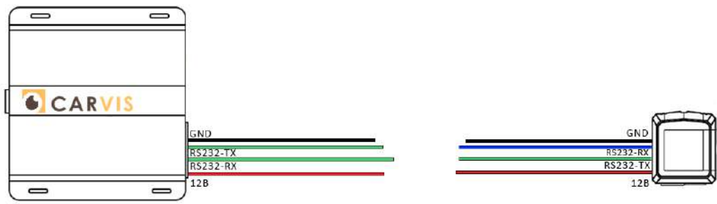
Рисунок 98 – Схема подключения регистратора к дисплею CARVIS CP-02
