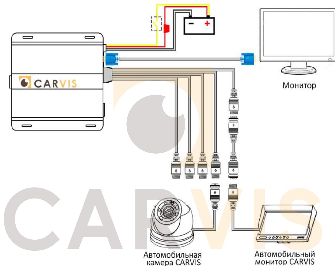
Рисунок 11 – Подключение питания
