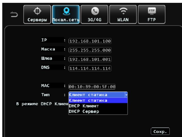
Рисунок 89 – Вкладка «Локал.сеть»
