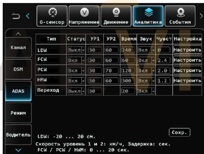
Рисунок 53 – Вкладка «ADAS»
