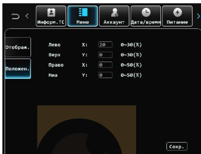
Рисунок 43 – Вкладка «Положение»
