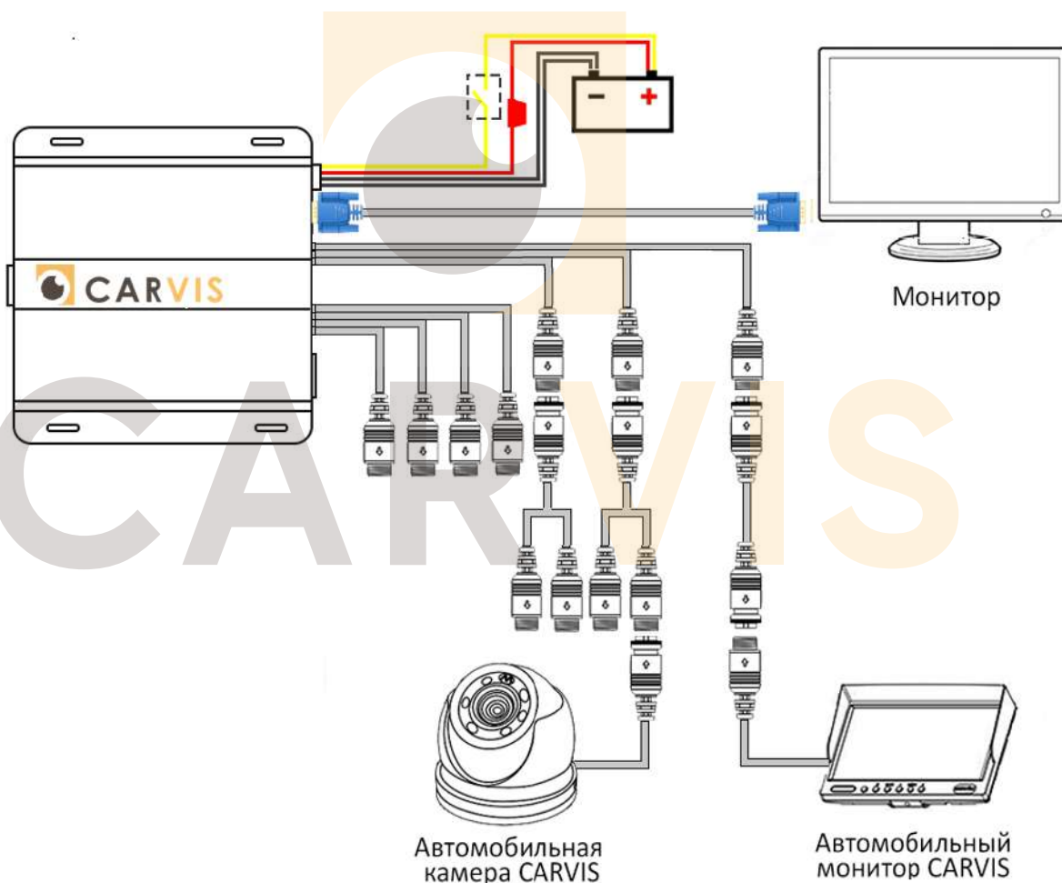
Рисунок 10 – Подключение питания
