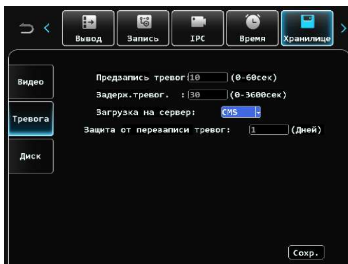
Рисунок 82 – Вкладка «Тревога»
