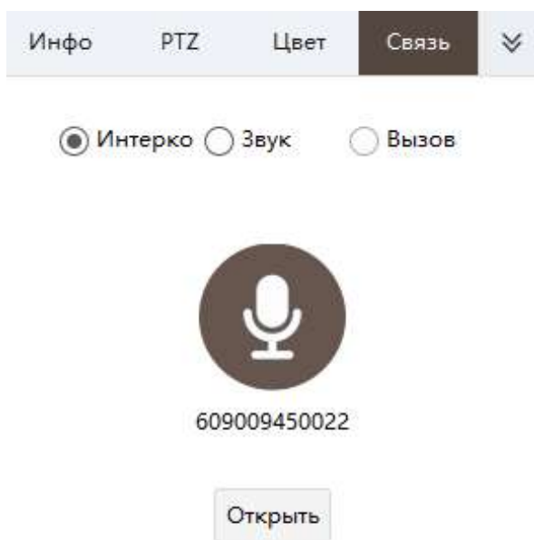
Рисунок 139 – Вкладка «Связь»
