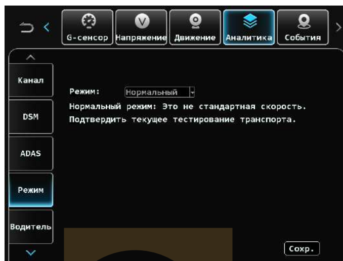
Рисунок 54 – Вкладка «Режим»
