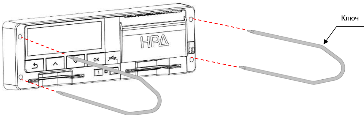
Рисунок 1. Извлечение тахографа
