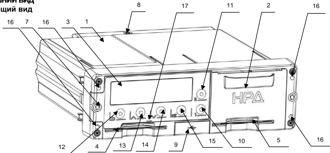
Рисунок 1. Вид спереди
