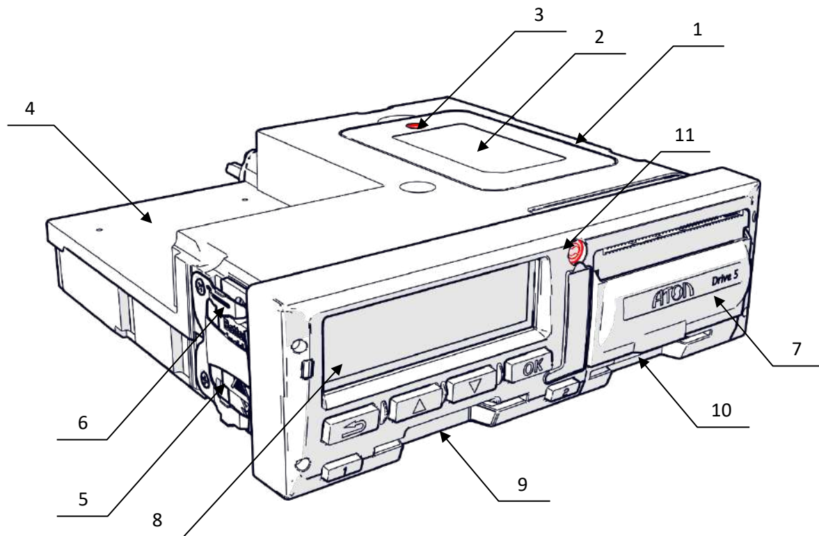
Рисунок 2. Внешний вид тахографа
