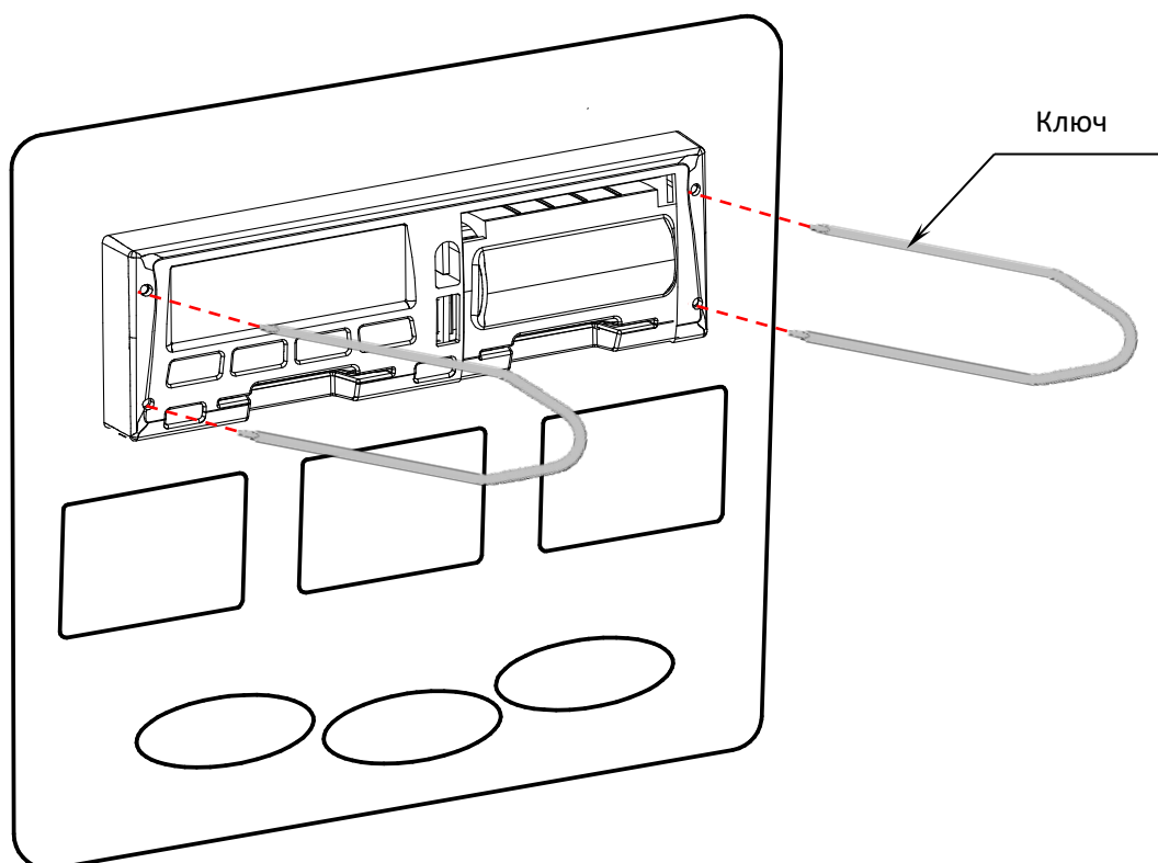
Рисунок 1. Извлечение тахографа
