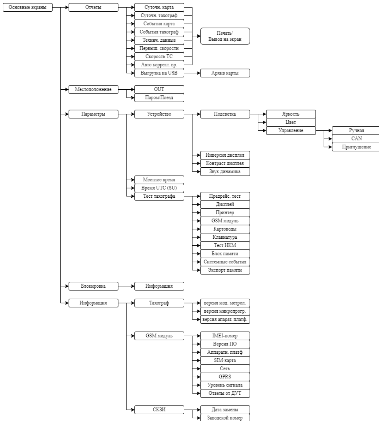
Рисунок 7. Структура меню рабочего режима
