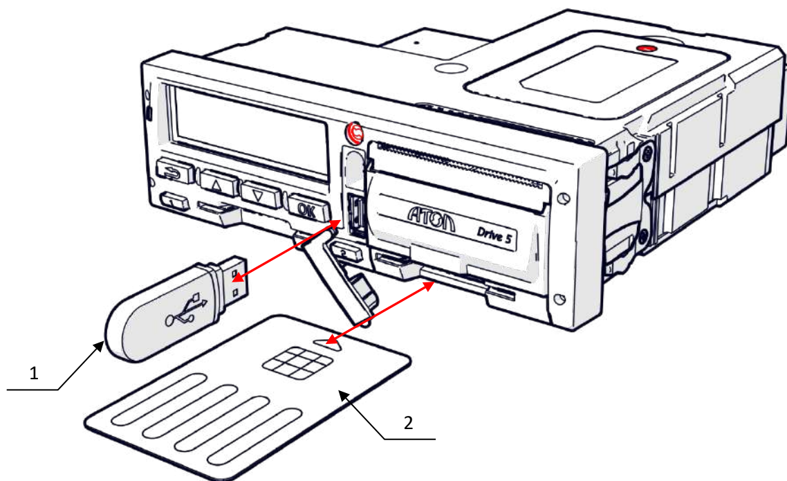
Рисунок 30. Выгрузка данных при помощи USB-накопителя
