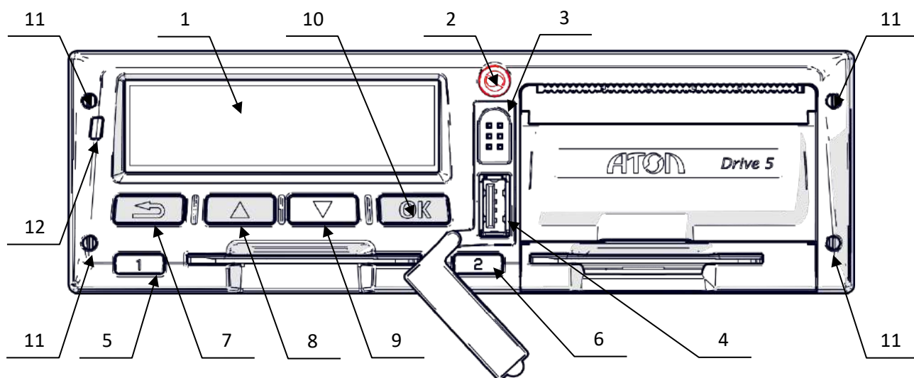
Рисунок 3. Вид спереди
