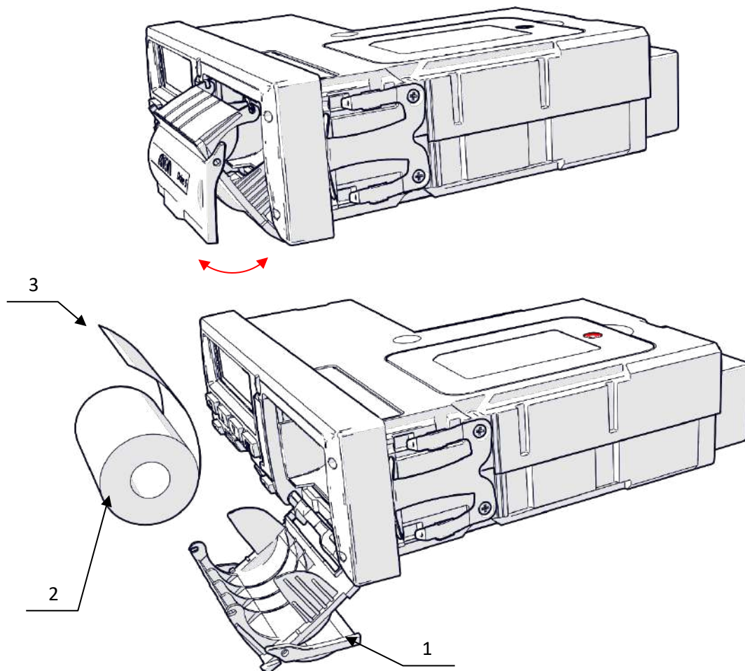
Рисунок 6. Установка бумаги
