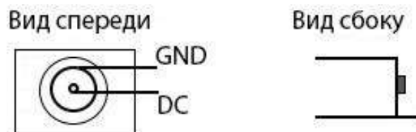
Рисунок 2 – Разъем питания
