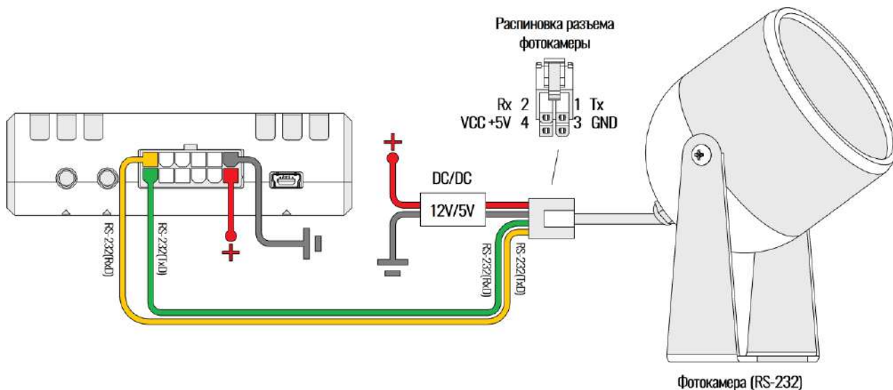
Рисунок 2.30 Подключение фотокамеры JC029F-Y01 с RS-232
