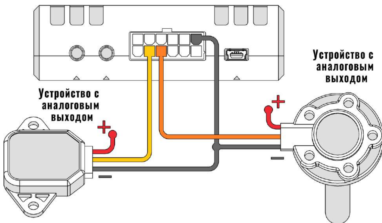
Рисунок 2.12 Подключение аналоговых источников
