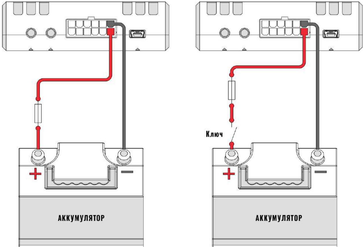
Рисунок 2.11 Подключение питания
