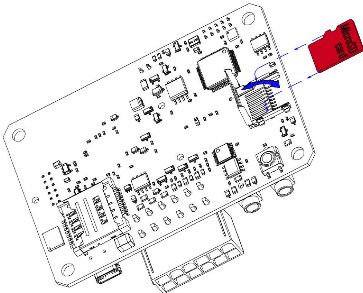
Рисунок 2.10 Установка microSD-карты
