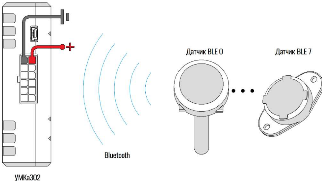
Рисунок 2.22 Подключение датчиков по BLE
