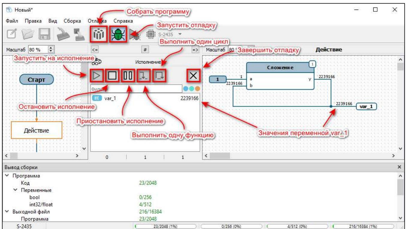
Рисунок 2.5 – Отладка программы
