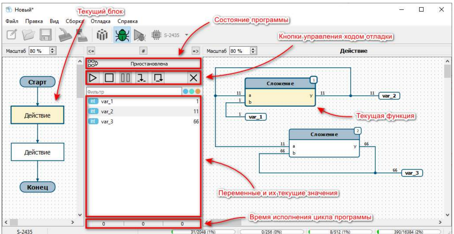
Рисунок 6.1 – Внешний вид редактора в режиме отладки
